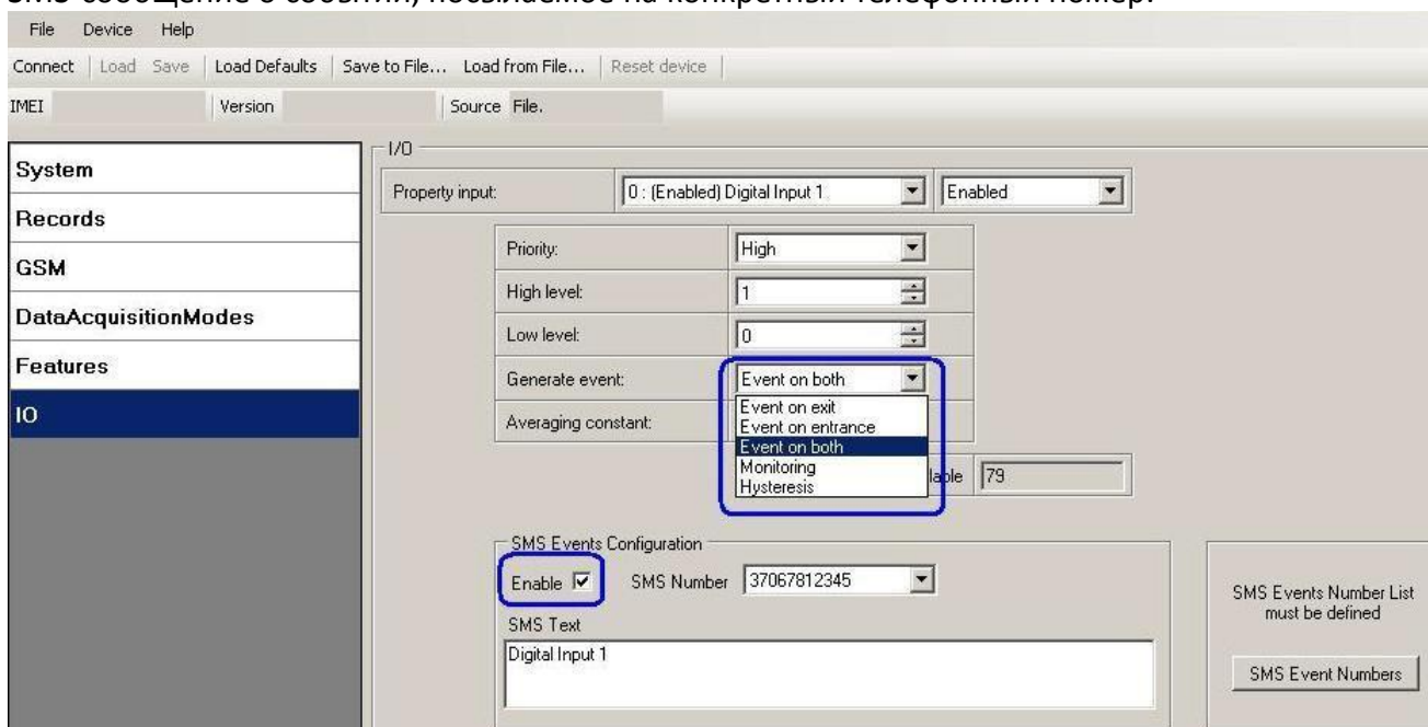
Рис. 33. Конфигурирование SMS-оповещений для событий I/O параметров.
