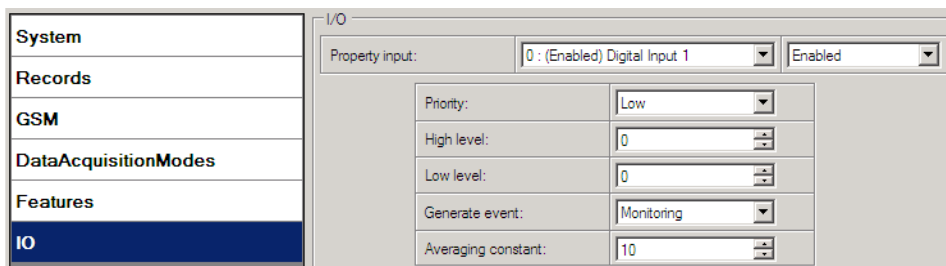
Рис. 34. Установки для I/O параметров.
