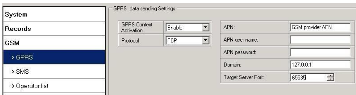
Рис. 14. Конфигурирование параметров GPRS
