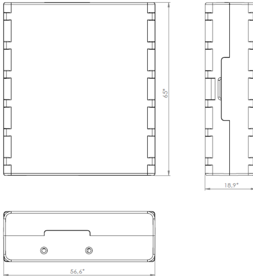
Рисунок 1. Внешний вид и размеры FM1111 (точность \pm 2\text{mm} )
