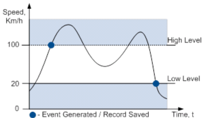
Рис. 38. Регистрация событий по принципу гистерезиса.
