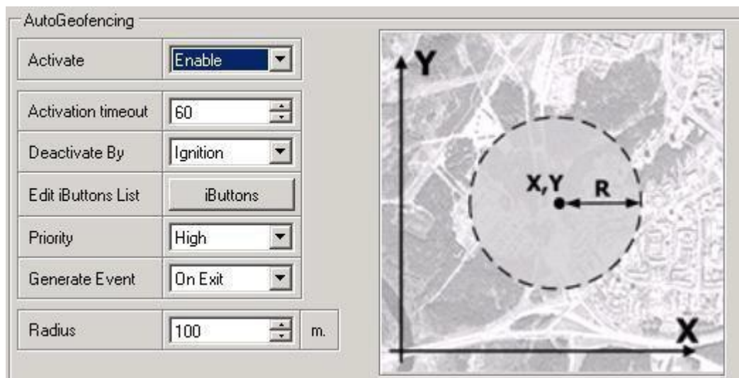
Рис. 26 Конфигурирование функции AutoGeofencing.
