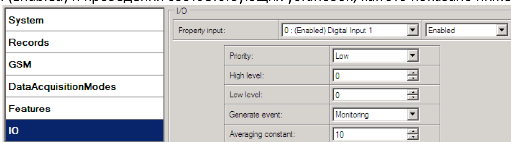
Рис. 42. Установки для параметров I/O.
