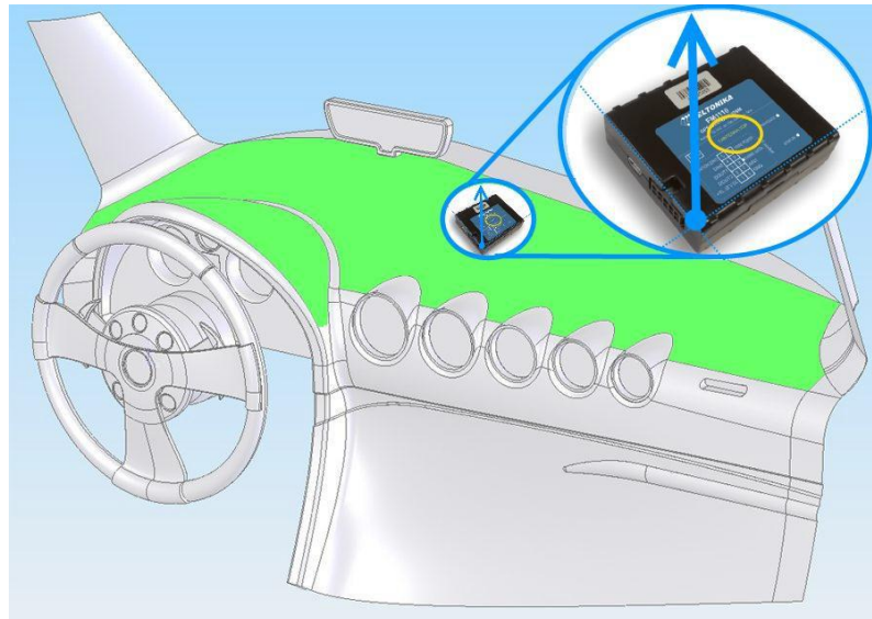
Рис. 40. Правильное размещение FM1111.
