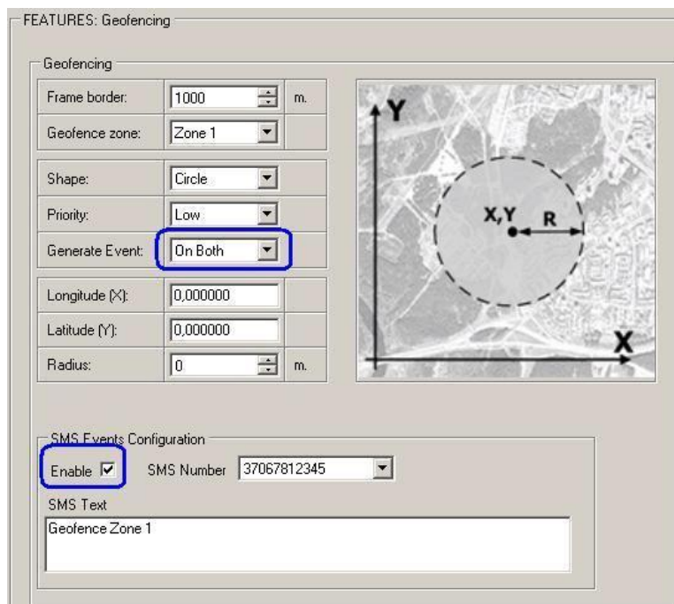
Рис. 31 Конфигурирование SMS-сообщения о событиях в геозоне.
