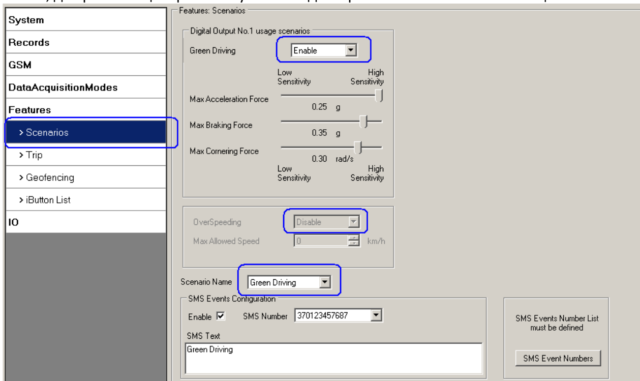
Рис. 29. Конфигурирование SMS оповещений о событиях в сценариях.
