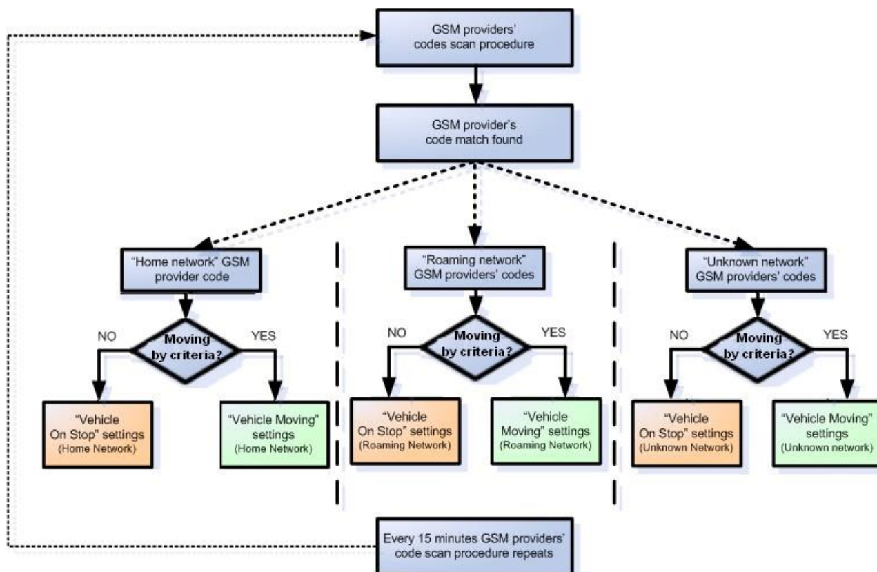
Рис. 17. Конфигурирование режимов регистрации данных.
