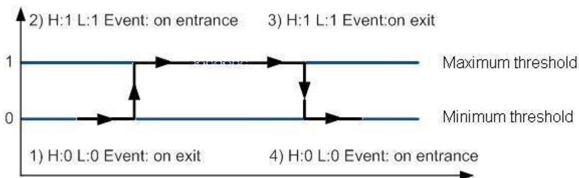
Рис. 36. Пример регистрации события для цифрового входа.
