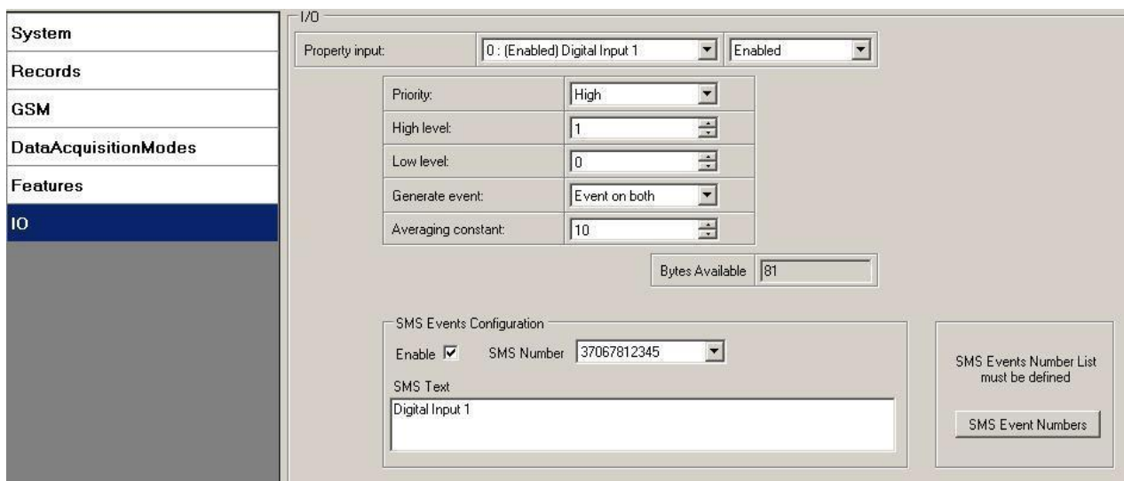
Рис. 28. Конфигурирование оповещения по SMS о событии на Digital Input 1.
