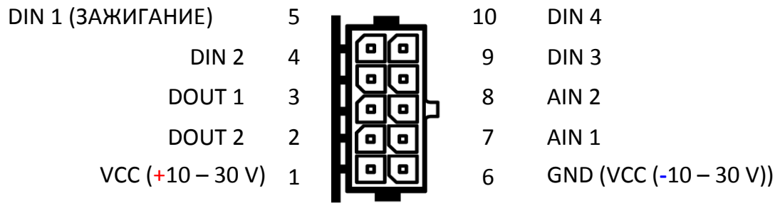
Рис. 5. Описание контактов разъема 2x5
