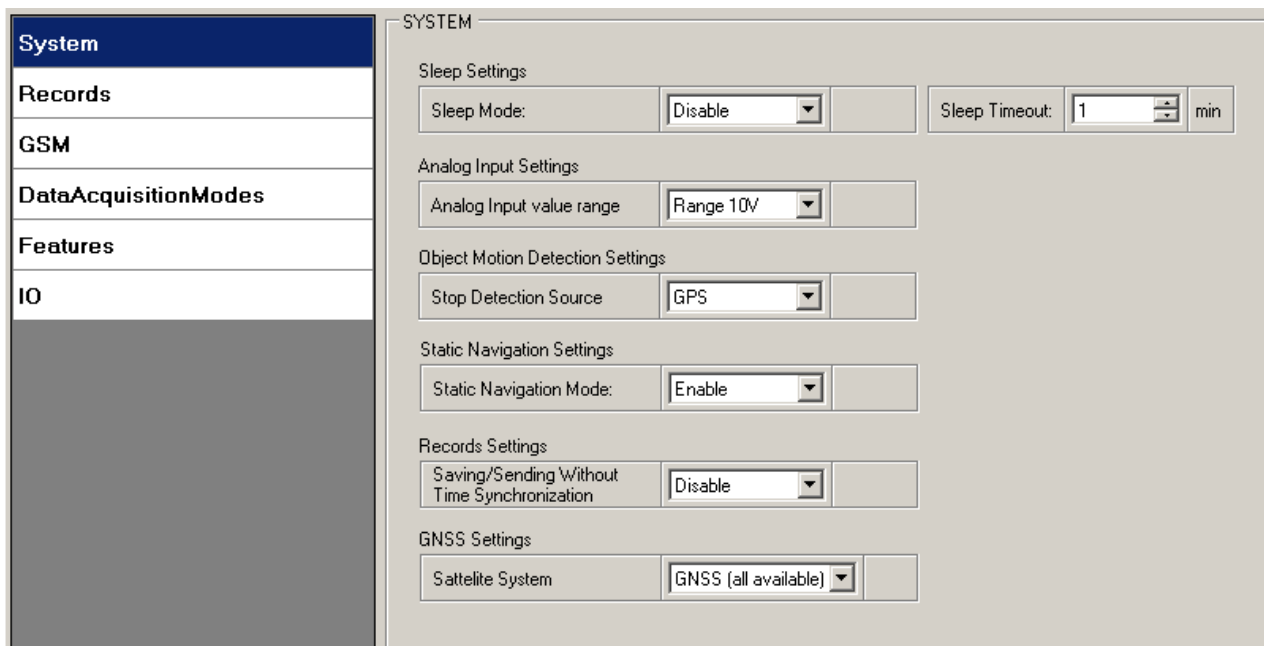
Рис. 12. Конфигурирование системных параметров
