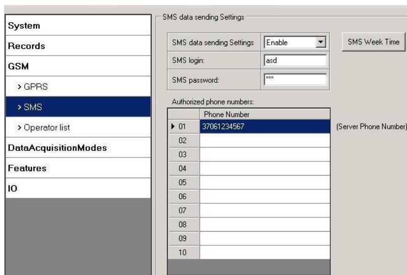
Рис. 15. Конфигурирование параметров SMS.
