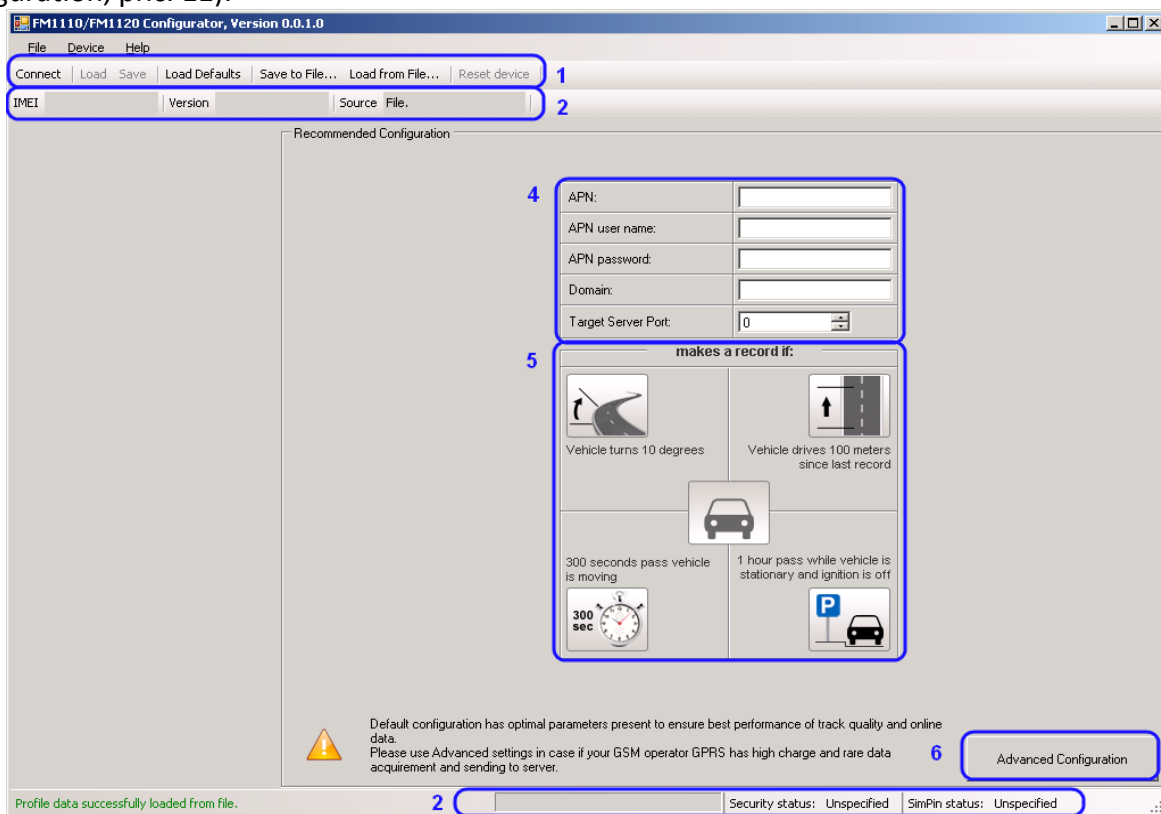
Рис. 10. Окно рекомендованного конфигурирования.
