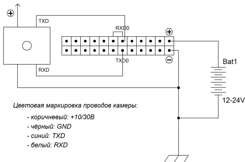
Рисунок 4. Схема подключения по протоколу RS232
