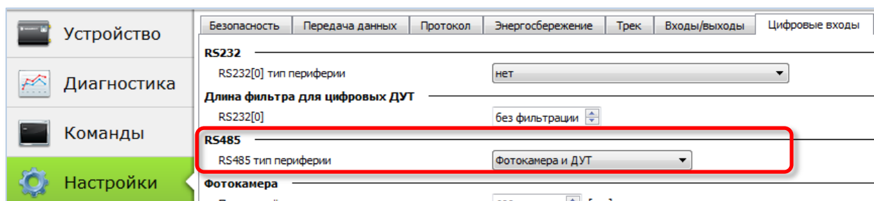
Рисунок 8. Настройка входа RS485 в Конфигураторе
