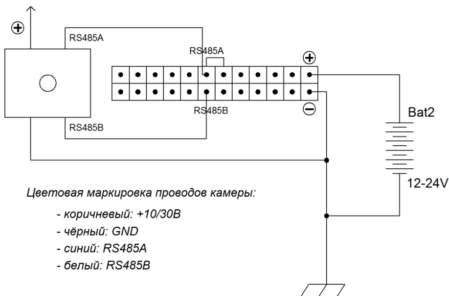
Рисунок 7. Схема подключения по протоколу RS485
