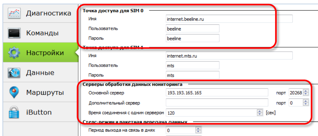
Рисунок 10. Пример настройки параметров сервера
